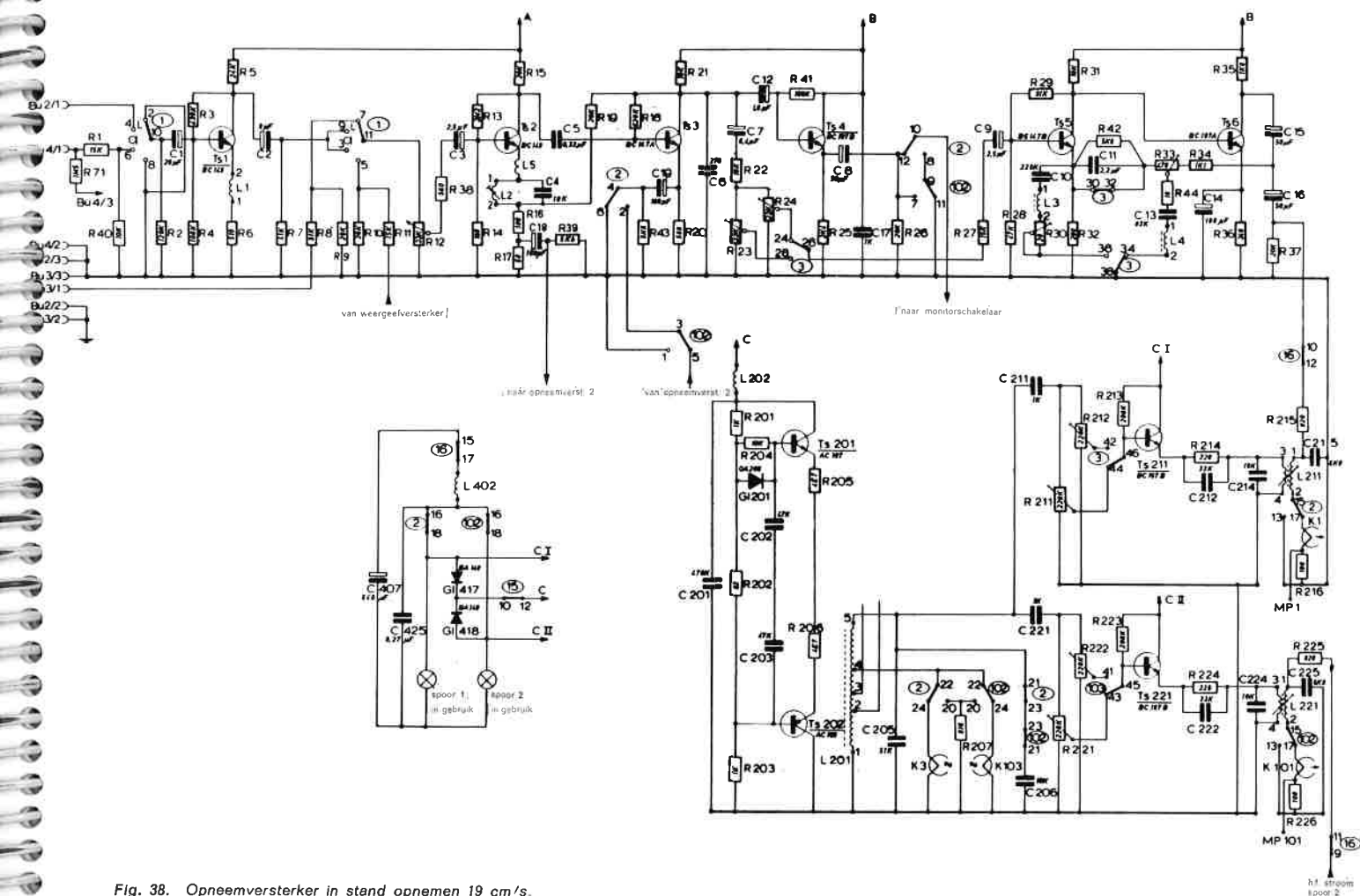
Fig. 38. Opneemversterker in stand opneemen 19 cm/s.
