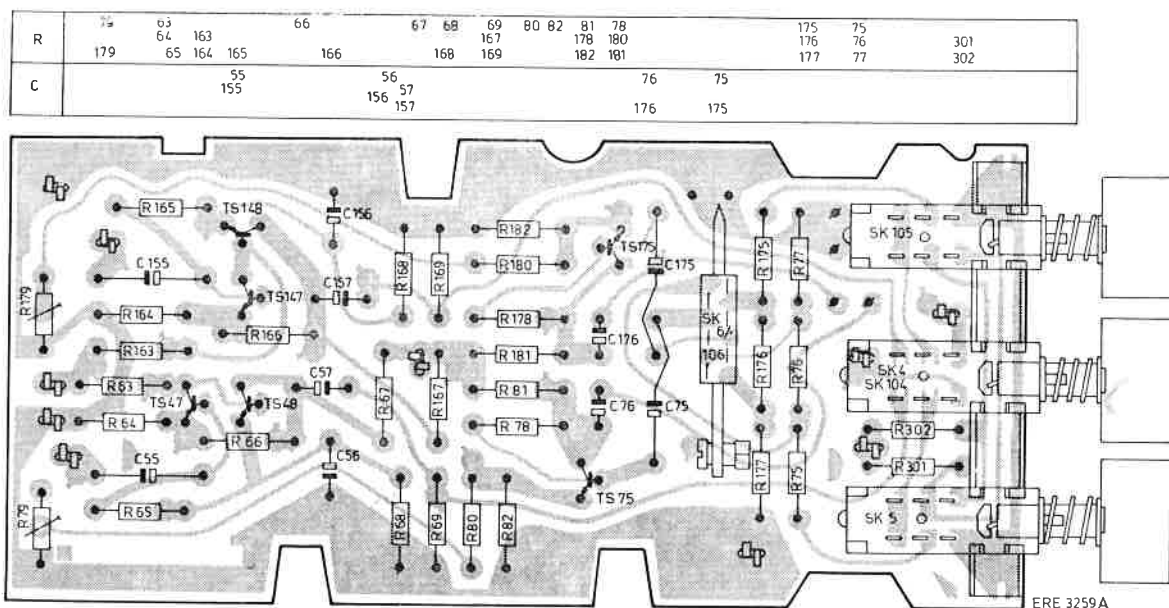
Fig. 33. Gecombineerde prent van eindtrap van opneemversterker en VU-meterversterker.
