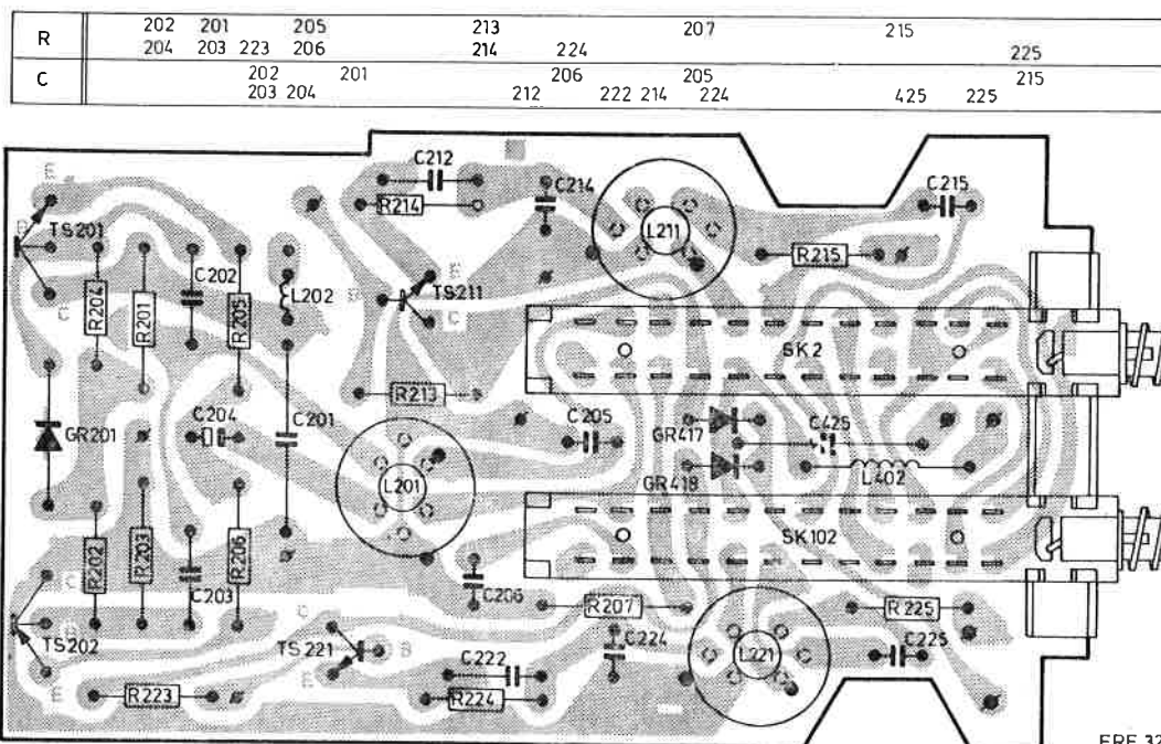
Fig. 33. Gecombineerde prent van eindtrap van opneemversterker en VU-meterversterker.
