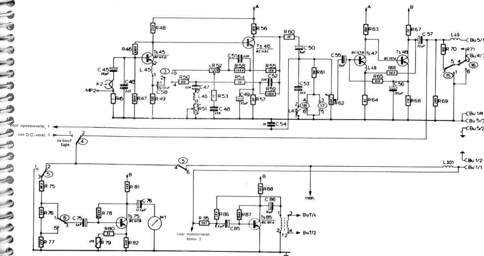
Fig. 39. Weergeefversterker in stand weergeven 19 cm/s
