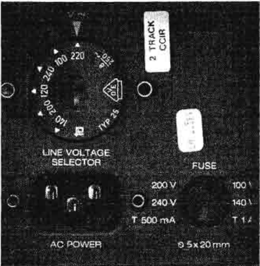
Sélecteur de tension
